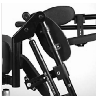
Fussstütze hochschwenkbar
